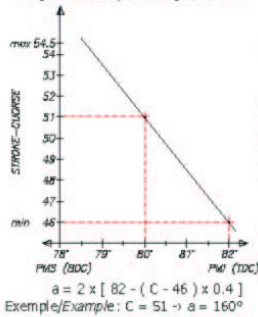
DIAGRAMME B / DIAGRAM B Diagramme de la lumière d'admission comparée avec la course Diagram of inlet port timing vs. stroke
