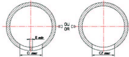
DIAGRAMME B / DIAGRAM B Diagramme de la lumière d'admission comparée avec la course Diagram of inlet port timing vs. stroke
