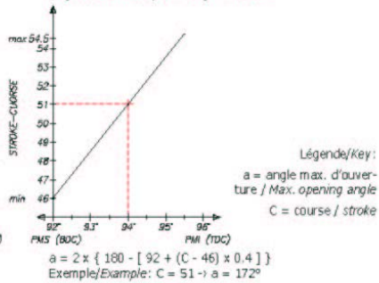
DIAGRAMME A / DIAGRAM A Diagr. de la lumière d'échappement comparée avec la course Diagram of exhaust port timing vs. stroke
